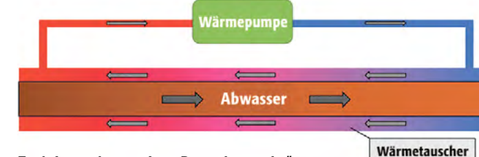
Funktionsschema eines Doppelmantelwärmetauschers, der Wärme aus KMS-Abwasser „macht“.
